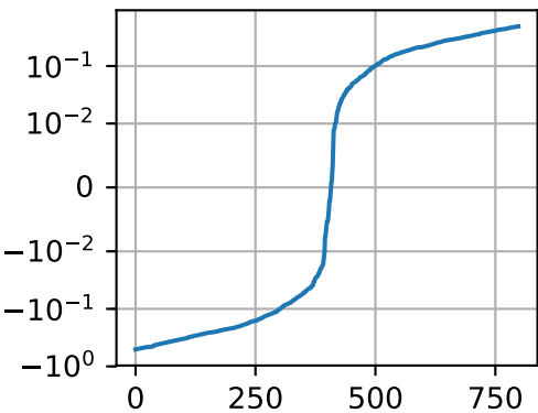
symlog
