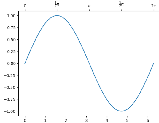
Fig. 55: Simple Axisline4
