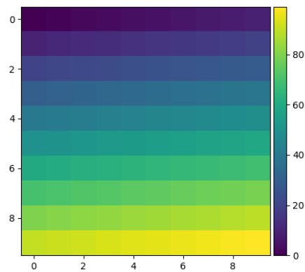
Fig. 52: Simple Colorbar
