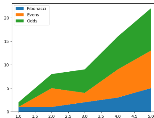
Fig. 22: Stackplot Demo2
