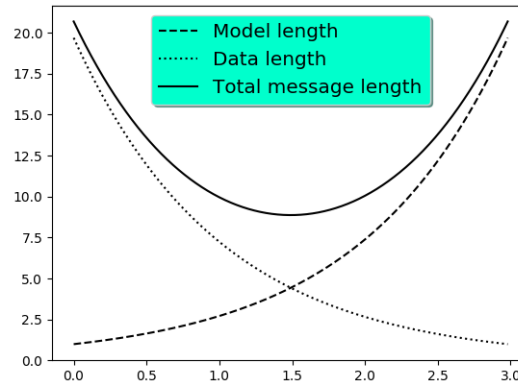
Fig. 19: Legend
