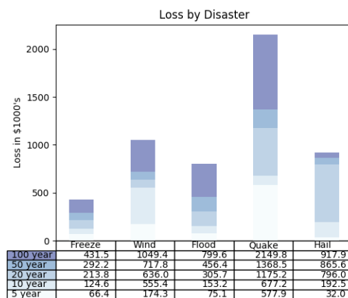
Fig. 12: Table Demo
