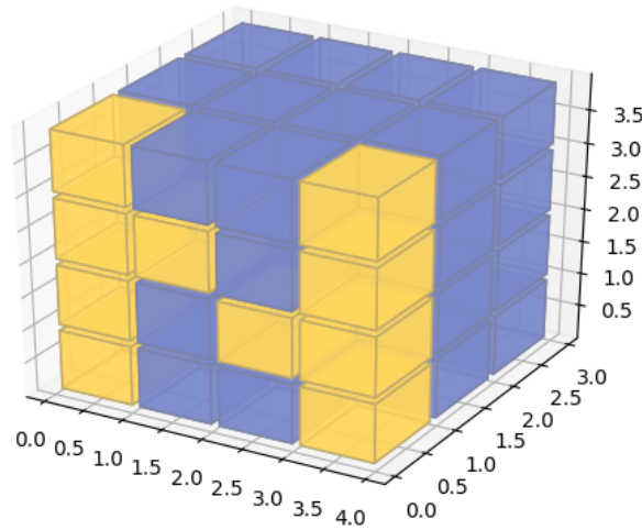
Fig. 31: Voxel Demo
