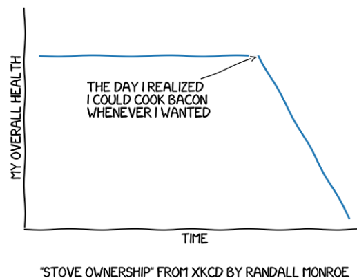
Fig. 18: Xkcd
