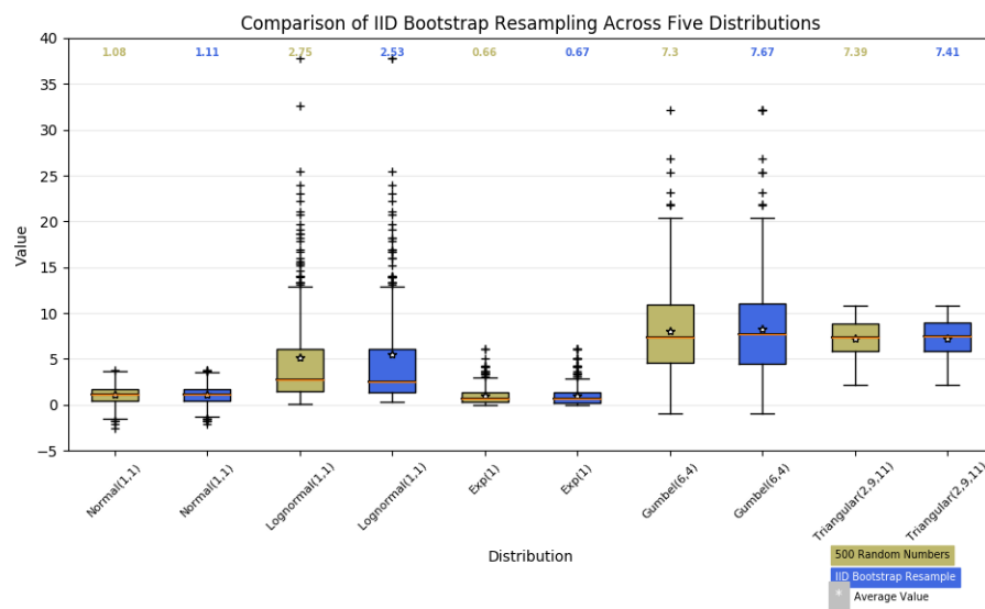
Fig. 14: Boxplot Demo3
