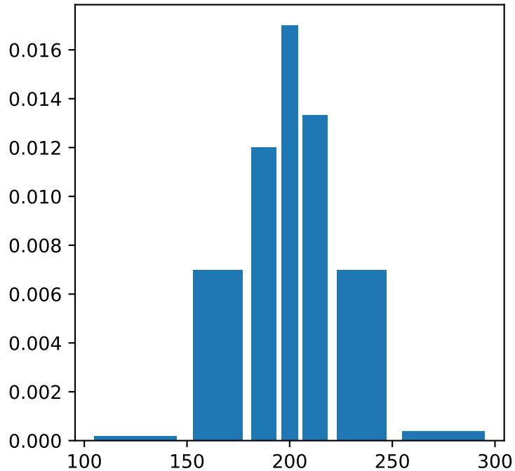
unequal bins
