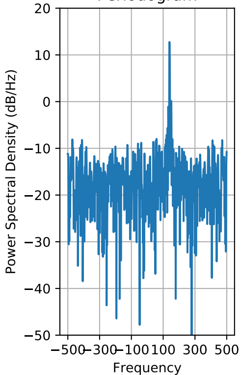
Periodogram
