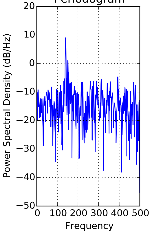
Periodogram
