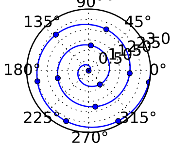
markevery=0.3
