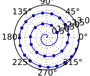
markevery=(0.45, 0.1)
