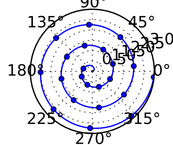
markevery=(30, 8)
