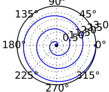
markevery=[0, -1]
