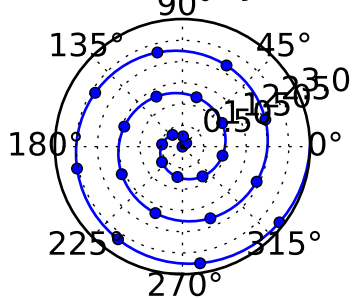
markevery=8
