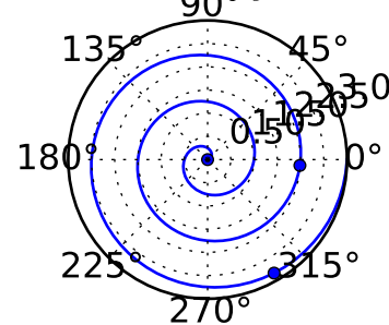
markevery=1.5
