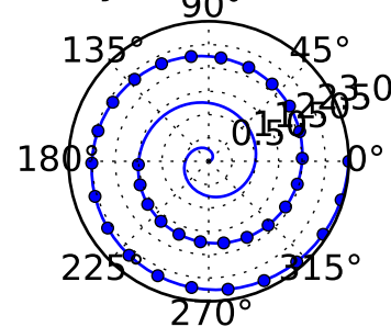
markevery=slice(100, 200, 3)
