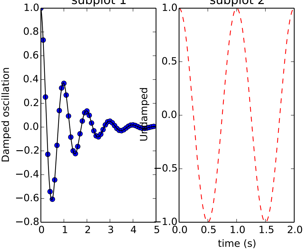
subplot 1
